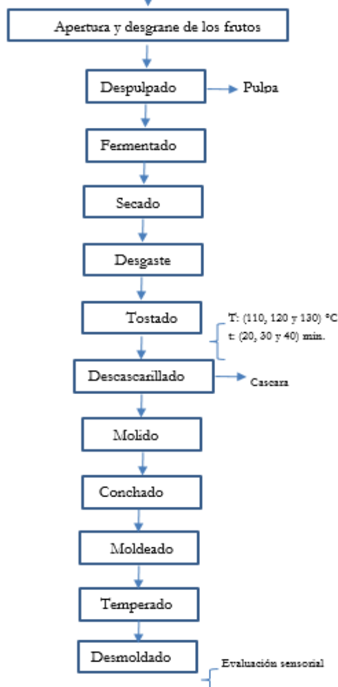
Figura 1. Flujograma de obtención de chocolate de copoazú
