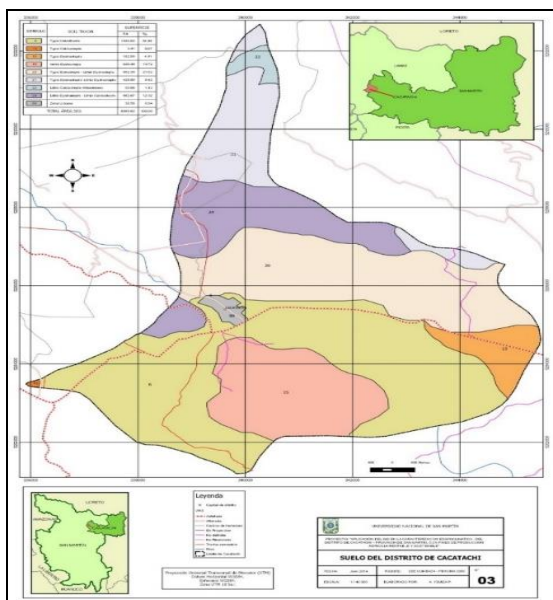
Figura 3. Características de los suelos del distrito de Cacatachi
